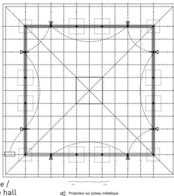
Plan de la halle sous toiture / Drawing of the hall below the roof
