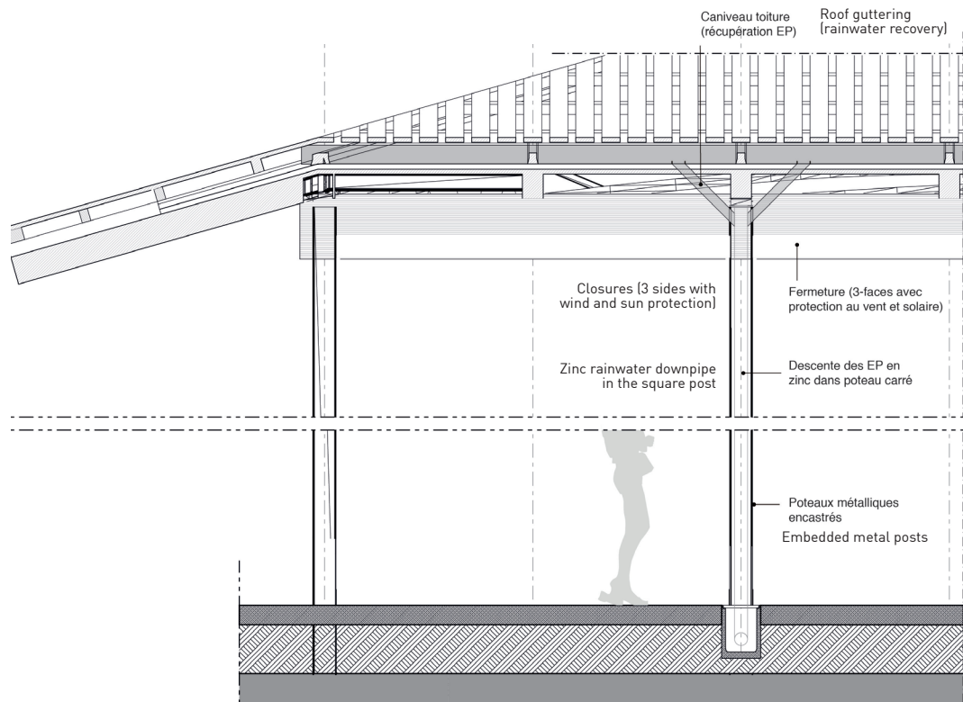
Coupe détail / Cross-section
